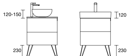
PIEDINI PER LAVABO D'APPOGGIO / VENETO ALTEZZA 230 MM
