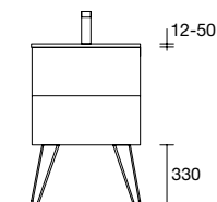
PIEDINI PER LAVABO INTEGRALE ALTEZZA 330 MM
